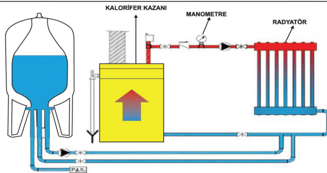
Bağlantı Şeması
